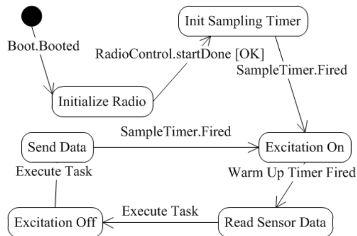
Fig. 3. SensIV State Diagram.
